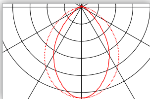
Diepe lichtbundel 60°
