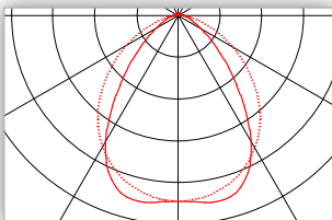
Gemiddelde lichtbundel 75°
